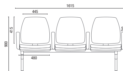
38010 Longarina Média
