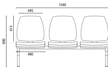
38010 Longarina Média
